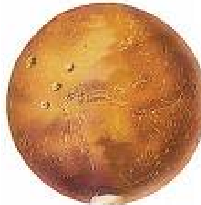
火星
